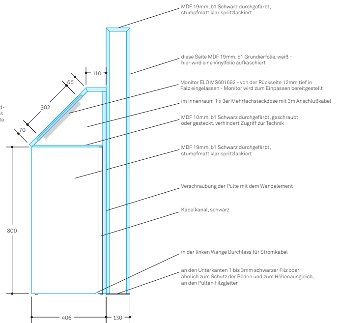
Schnitt A-A
