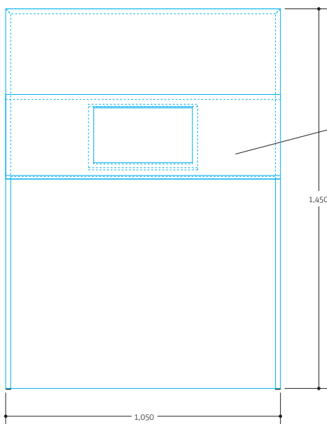
Ansicht
